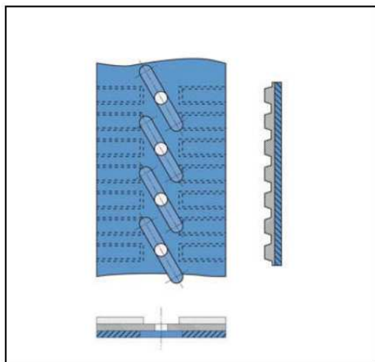
Typ B: 46 otworów z rowkiem, lewy
